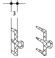
A-GS-240 (AE240) E Gasket
