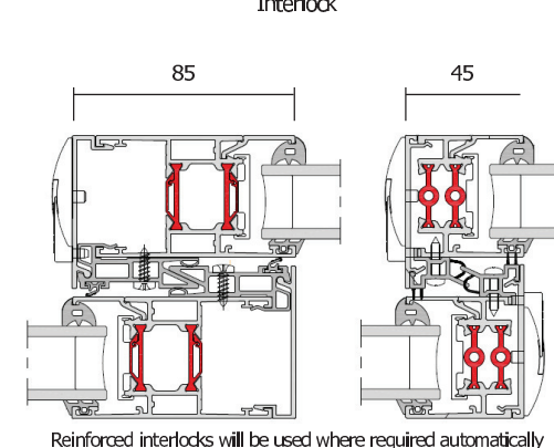
Interlock
